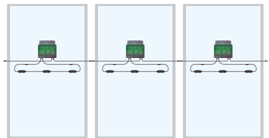
一拖一智能外挂 HCPO1-600 External Optimizer HCPO1-600
